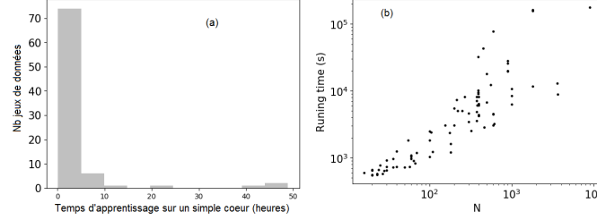
FIG. 5 – (a) Distribution des temps d'apprentissage (en heures) ; (b) temps d'apprentissage (en secondes) pour chaque jeu de données en fonction de la taille de l'ensemble d'apprentissage, N (échelle logarithme).
